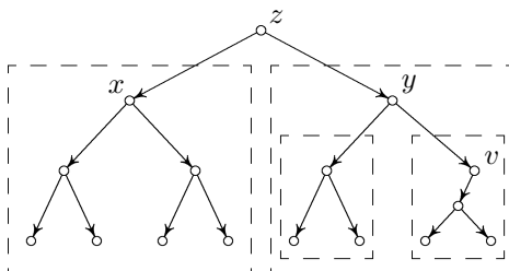
Obrázek 8.8: Binární kořenový strom a podstromy vrcholů z a y .
